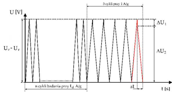
Rys. 3. Przebieg napięcia na zaciskach superkondensatora w pomiarach rozkładu temperatury [5].
