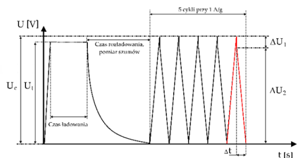
Rys. 4. Przebieg napięcia na zaciskach superkondensatora przy pomiarach szumów [12].
