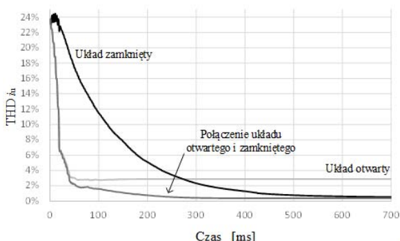
Rys.11. Zależność wartości współczynnika THD_u w funkcji czasu
