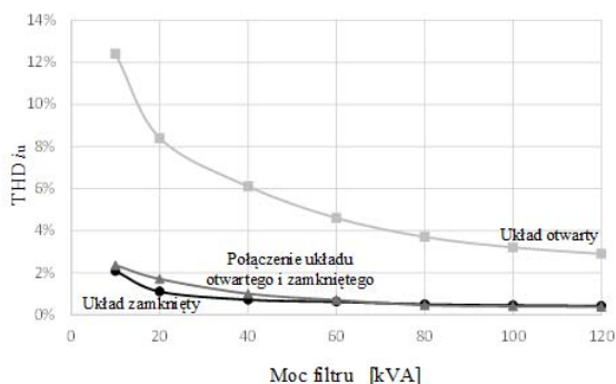
Rys.10. Zależność wartości współczynnika THD_u w funkcji mocy z jaką pracuje filtr (moc znamionowa filtra wynosi 120 kVA)
