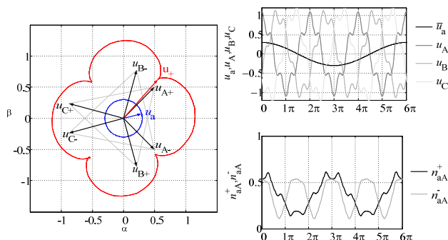
Rys.4. Synteza wektora wyjściowego: u_a wektor referencyjny, u_{A+} , u_{B+} , u_{C+} wektory wejściowe wirujące przeciwnie do wskazówek zegara, u_{A-} , u_{B-} , u_{C-} wektory wejściowe wirujące zgodnie ze wskazówkami zegara, n_{aA}^+ , n_{aA}^- współczynniki wypełnień, u_a wektor przestrzenny napięć wejściowych (jednostki względne).
